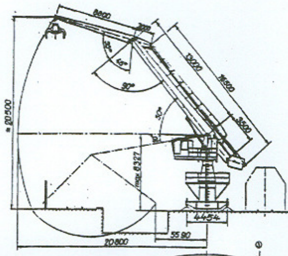
Zeichnung: Balance - Kran
